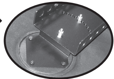
Vue du dessous avec boulons de montage en place.
