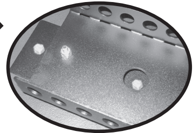
Vue du dessus avec boulons de la quincaillerie en place
