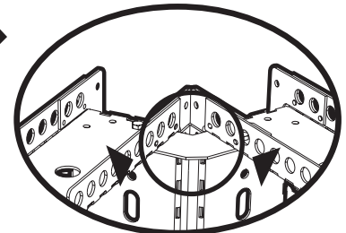
Placez les adaptateurs pour disposition circulaire NXF35A entre les quincailleries NXF35U – Vue du dessus de l'adaptateur –
