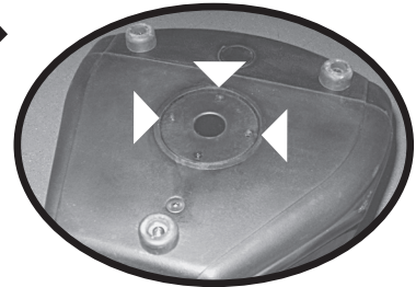
Vue du dessous exposant les boulons qui doivent être enlevés.
